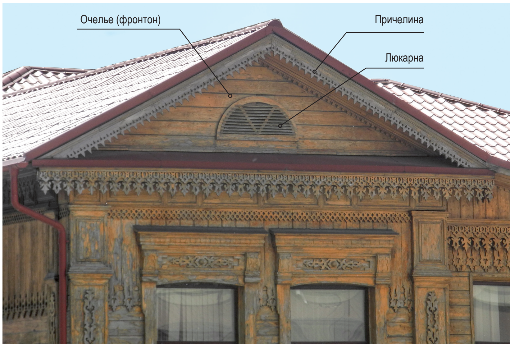
фрагмент северного фасада
