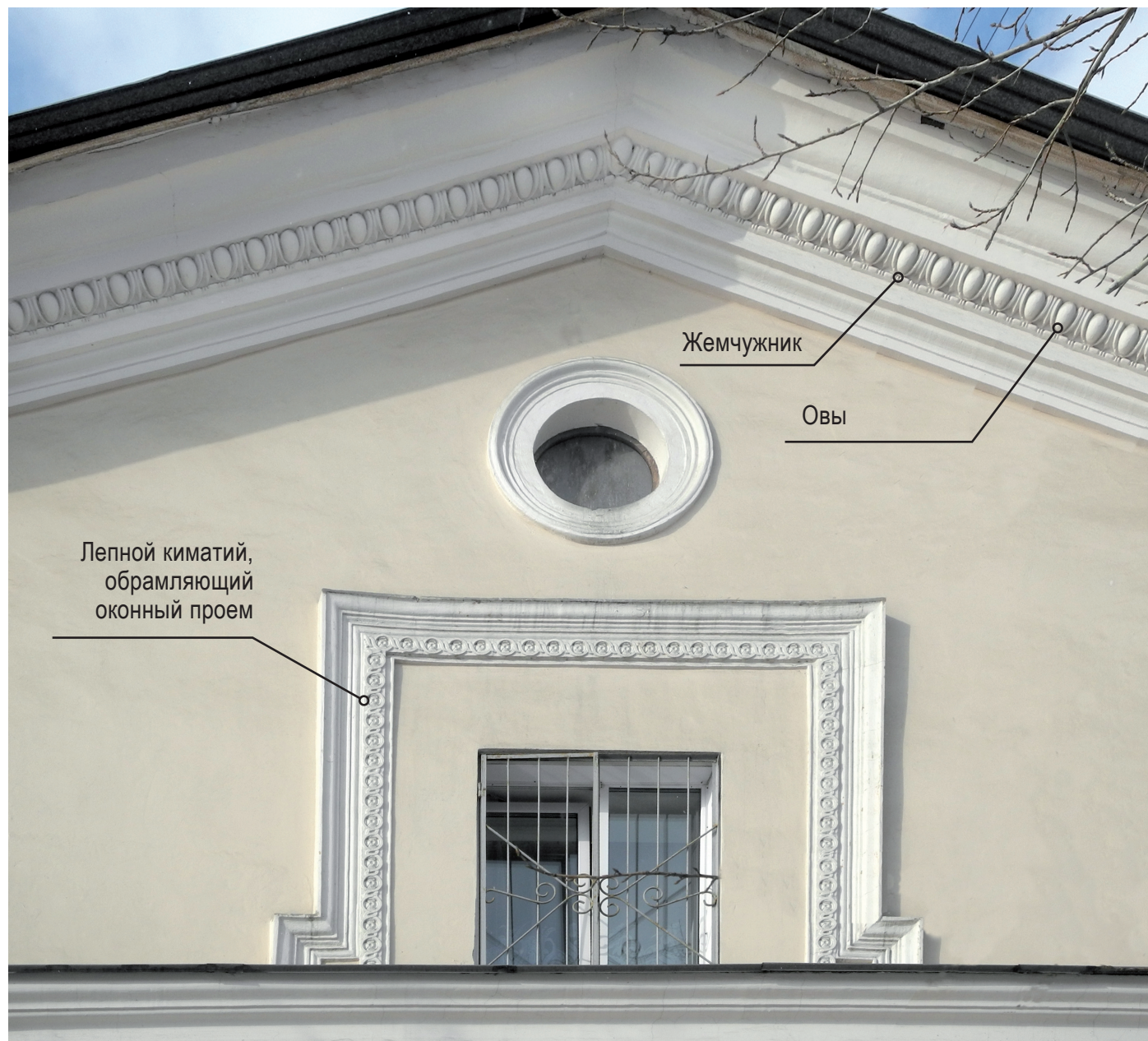
Фрагмент щипца
